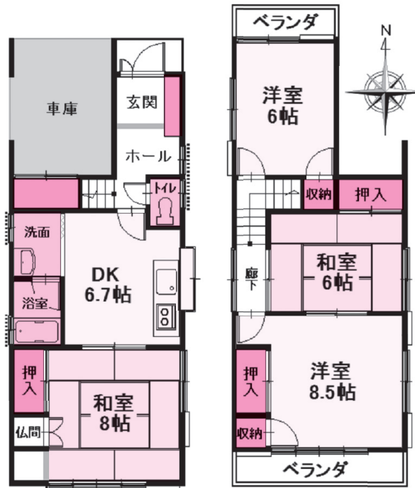
1F 平面図
